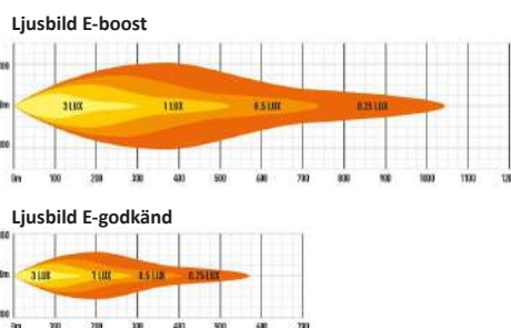
LINEAR 18 ELITE MED LOW BEAM ASSIST 159208
